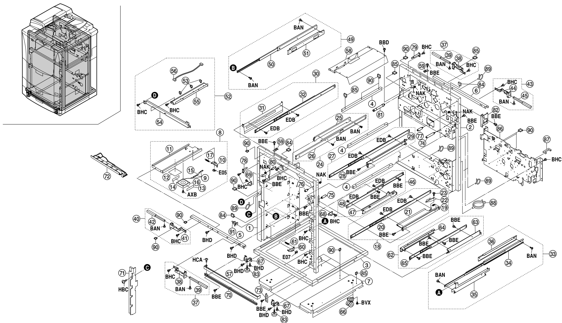
FIG. 2 FRAMES
