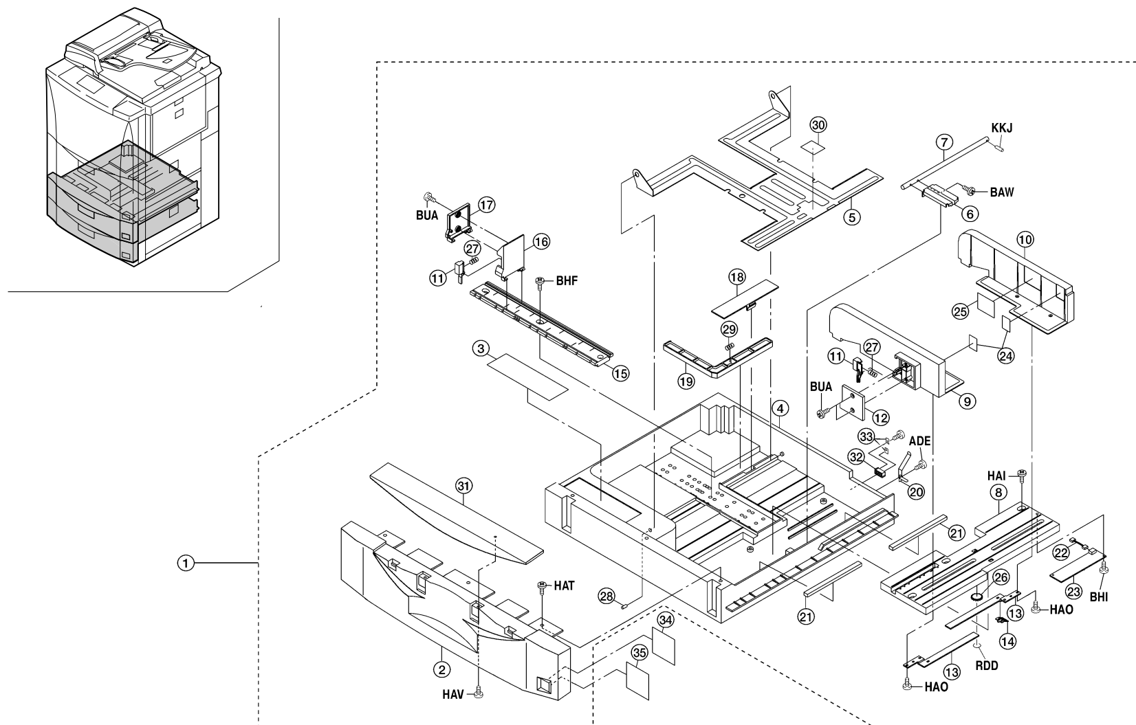
FIG. 3 CASSETTE(120V)
